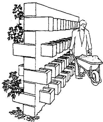
Figura 2.7 En Botswana, el Dr. Gus Nilsson ha desarrollado un sistema de producción hortícola intensivo para zonas tropicales secas, basado en paredes construidas con bloques prefabricados (también véase figura 5.3).
